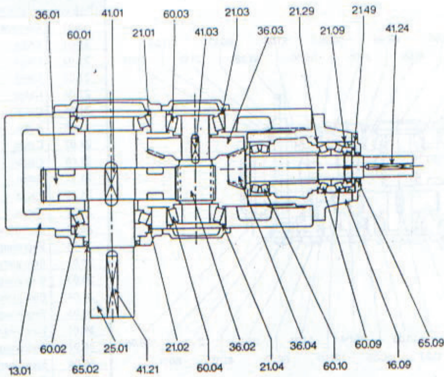
Fig. 7 - Eixos em Ângulo Reto Horizontal - Redução Dupla
