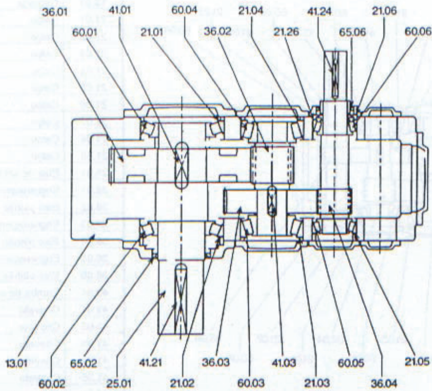
Fig. 1 - Eixos Paralelos Horizontal - Redução Dupla
