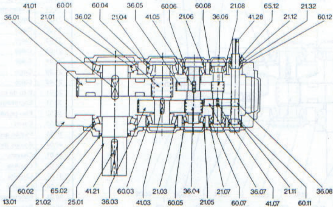
Fig. 5 - Eixos Paralelos Horizontal - Redução Quádrupla
