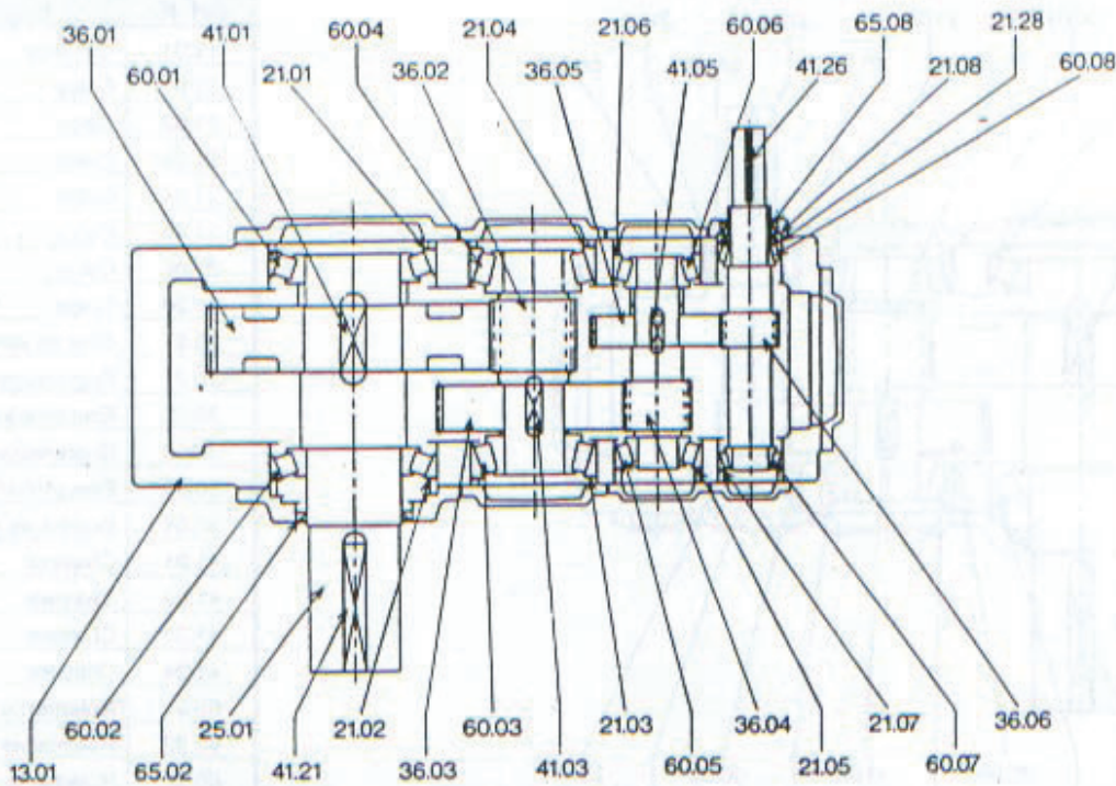
Fig. 3 - Eixos Paralelos Horizontal - Redução Tripla
