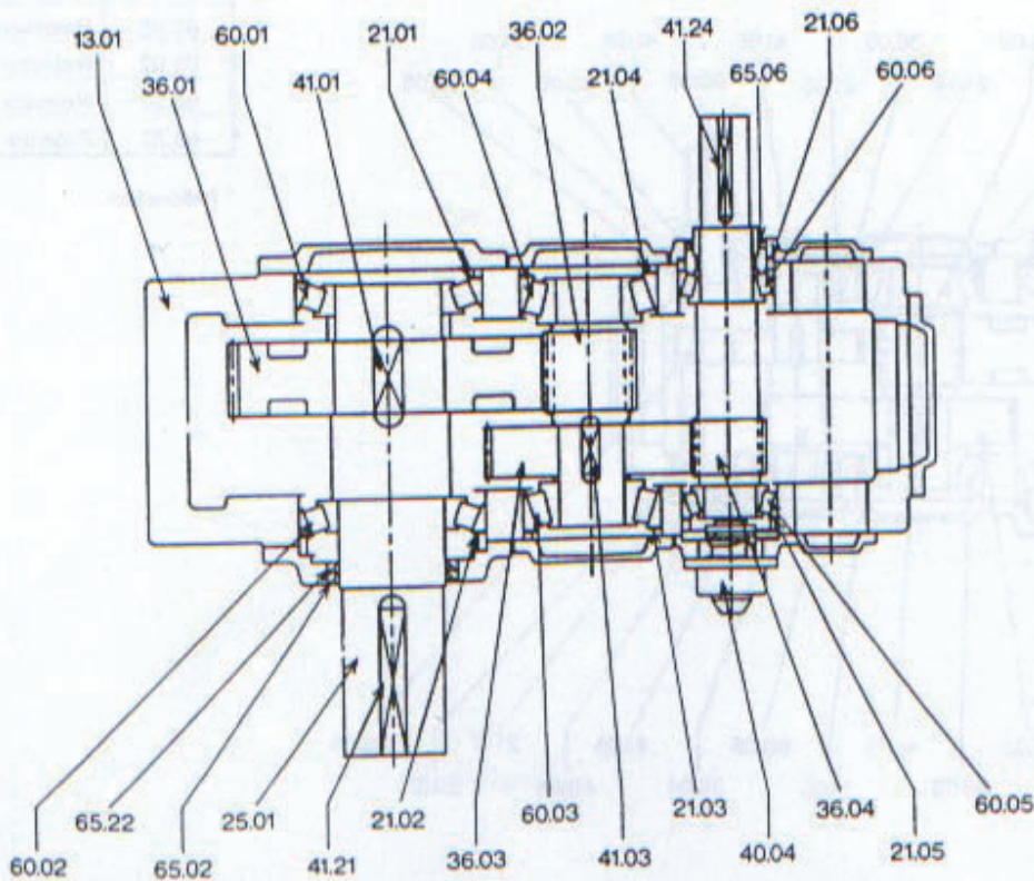
Fig. 2 - Eixos Paralelos Vertical - Redução Dupla
